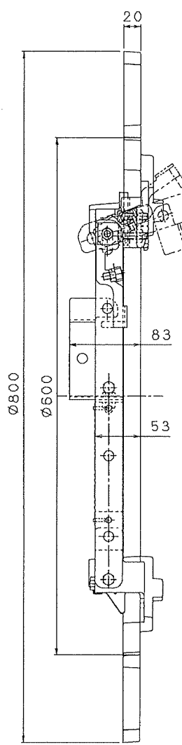
A-A断面図
